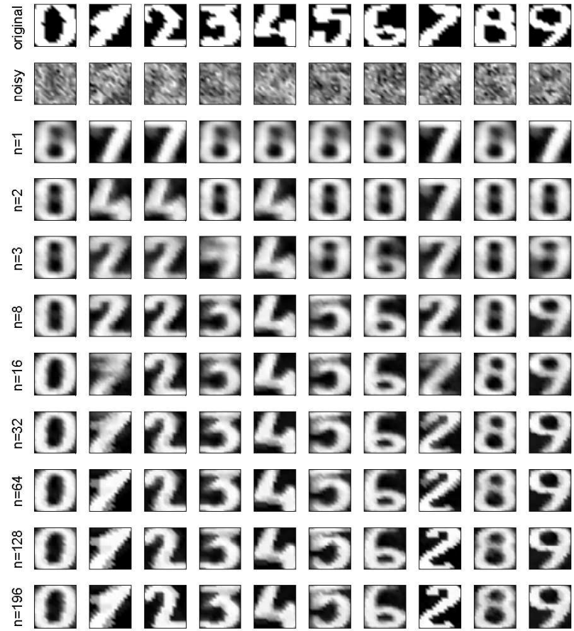
kernel PCA (RBF kernel)
