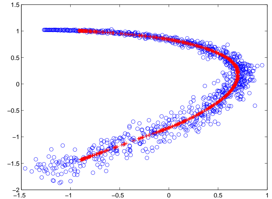
kernel PCA (RBF kernel)
